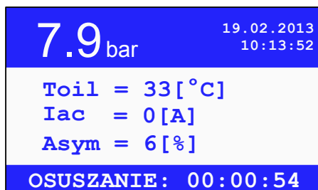
Rysunek 9: Widok ekranu z włączoną funkcją osuszania MS-485
