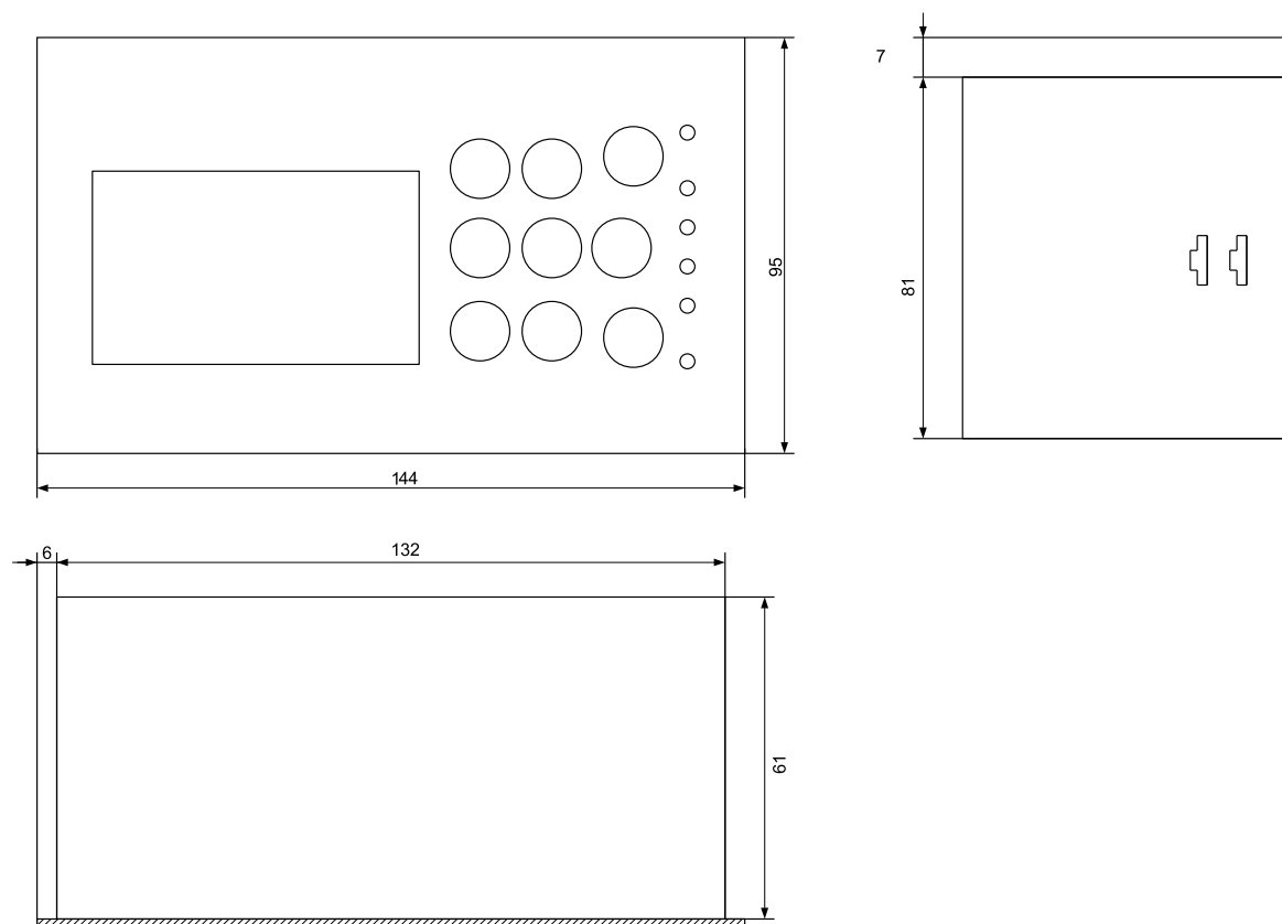
Rysunek 12: Rysunek obudowy sterownika MS-485
