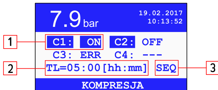
Rysunek 6: Widok menu pracy sieciowej
