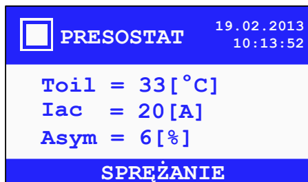
Rysunek 10: Widok ekranu z włączonym presostatem MS-485
