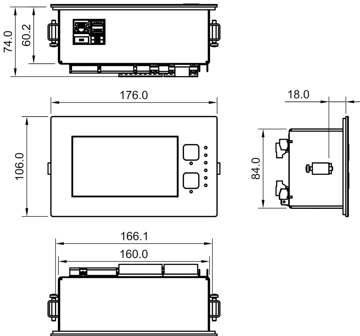
Rysunek 4: Rysunek obudowy sterownika XAIR Expert
