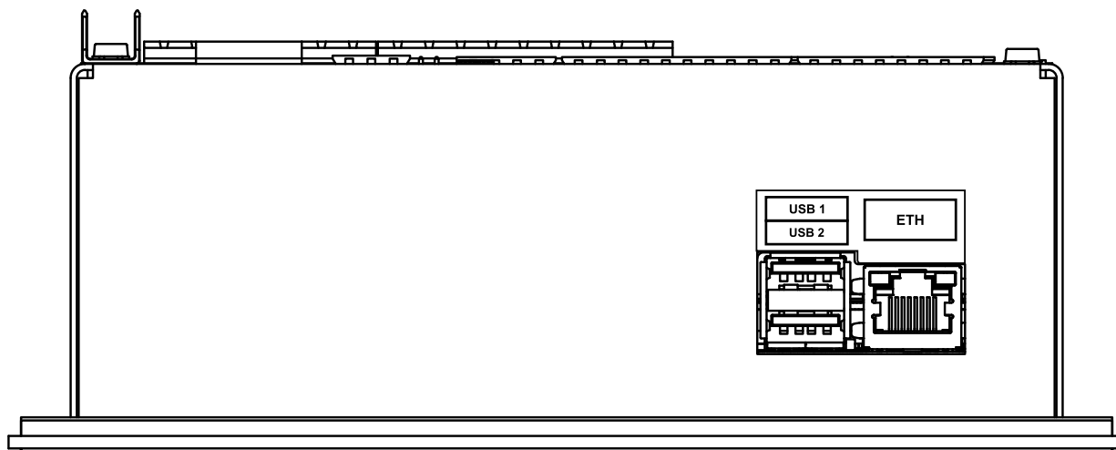
Rysunek 3: Złącza komunikacyjne sterownika XAIR Expert (spód obudowy)
