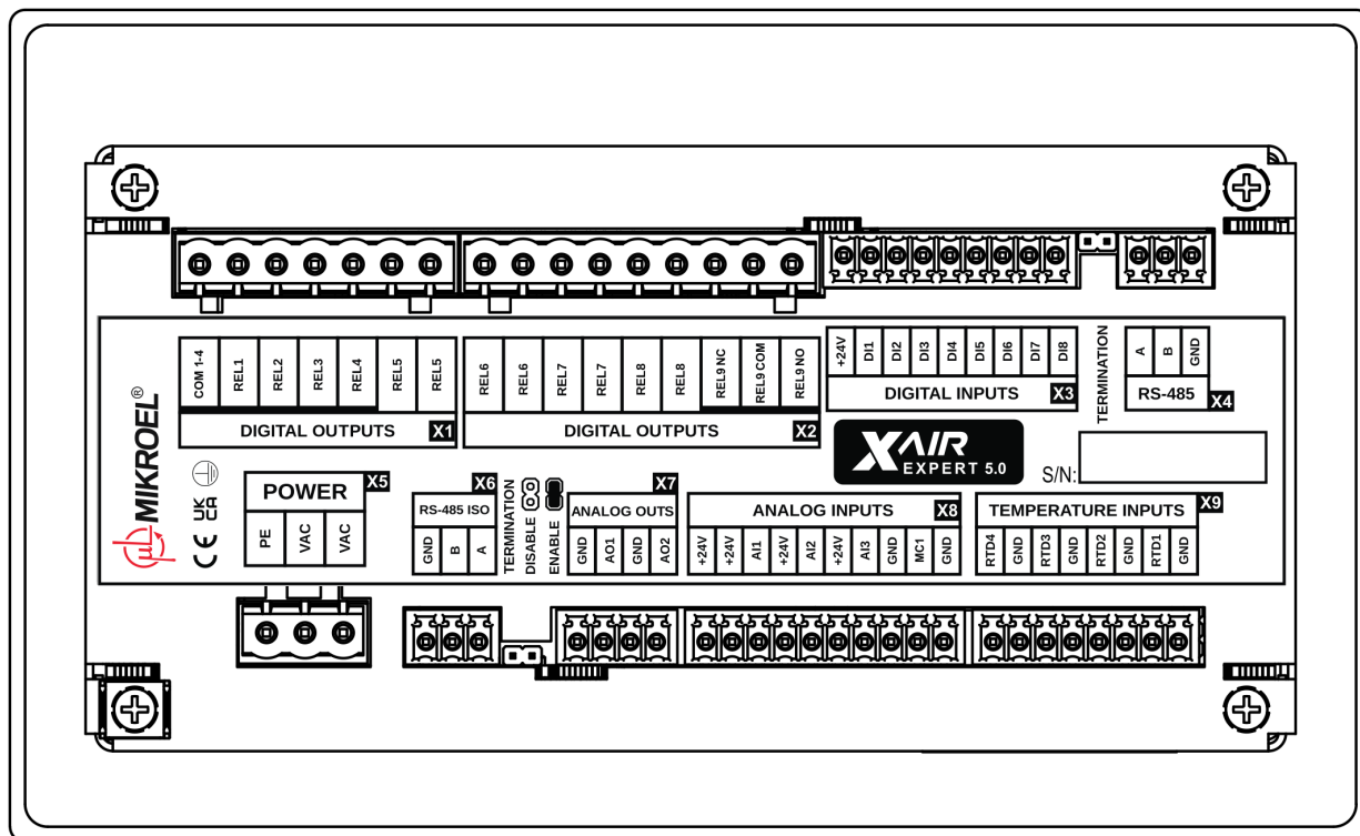
Rysunek 2: Wyprowadzenia elektryczne sterownika XAIR Expert (tylna ścianka obudowy)
