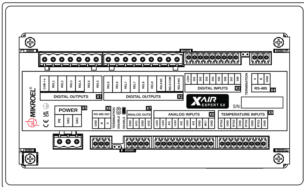
Рис. 2: Электрические соединения контроллера XAIR Expert
