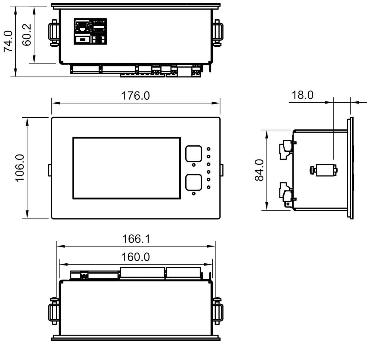
Рис. 4: Чертеж корпуса контроллера XAIR Expert
