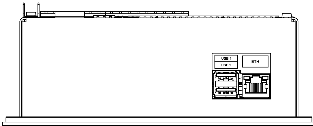
Рис. 3: Коммуникационные разъемы контроллера XAIR Expert (дно корпуса)
