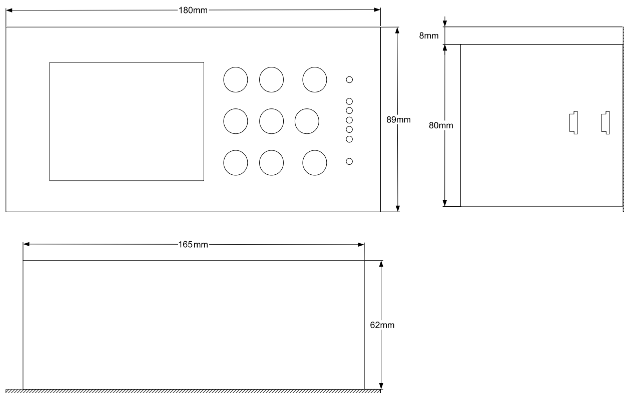
Rysunek 15: Rysunek obudowy sterownika MS-887VFD
