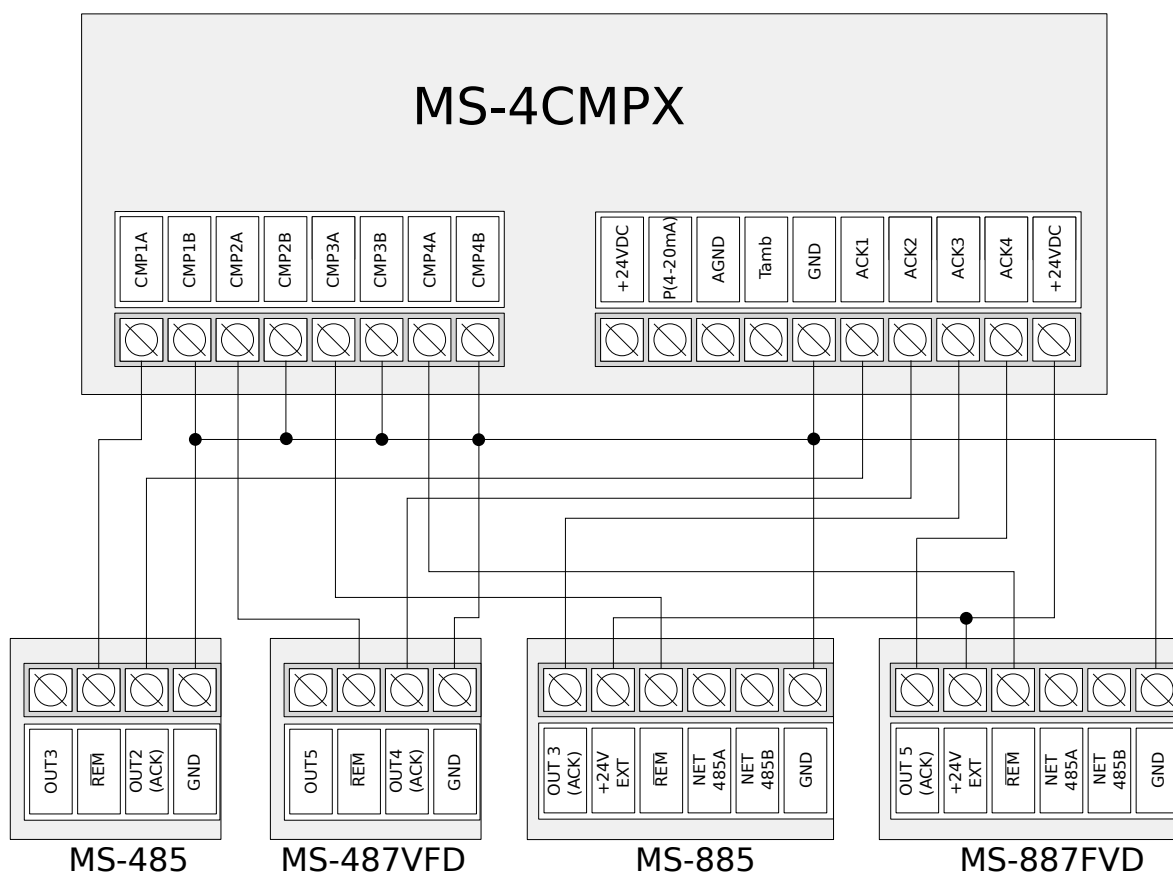
Rysunek 8: Schemat podłączenia sterownika
