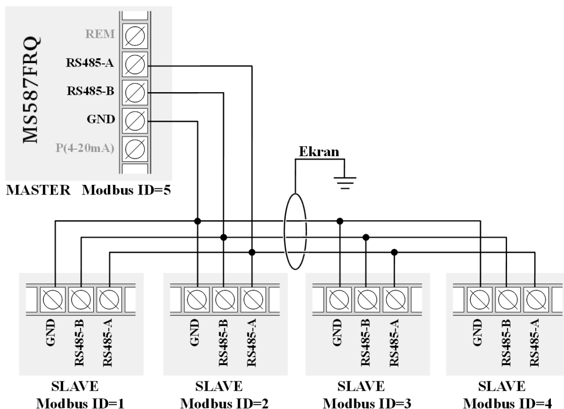
Rysunek 10: Schemat połączenia sterowników przez interfejs RS485
