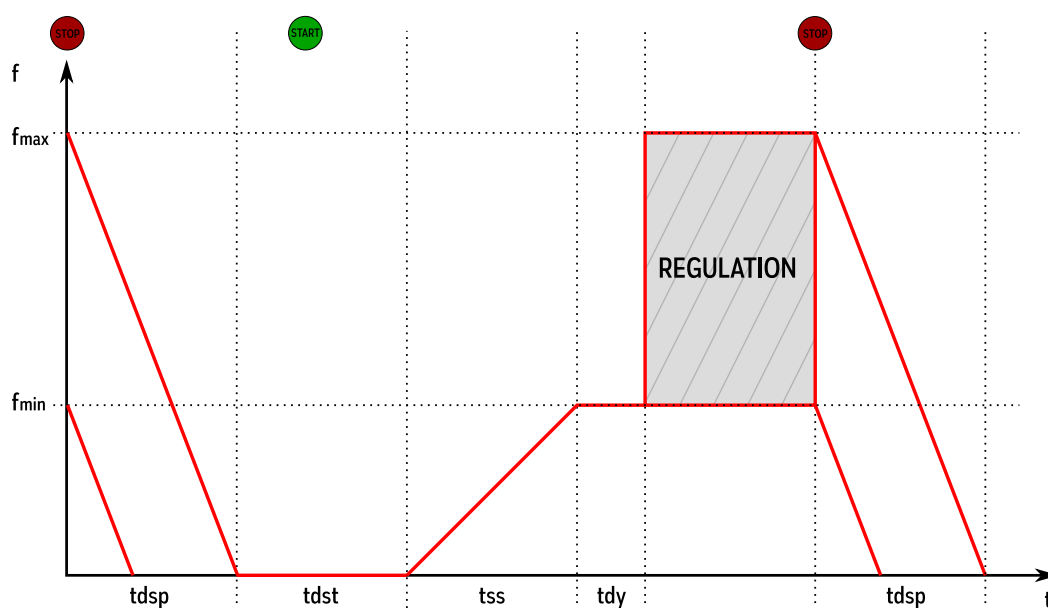
Rysunek 5: Zależności czasowe sterowania częstotliwością silnika
