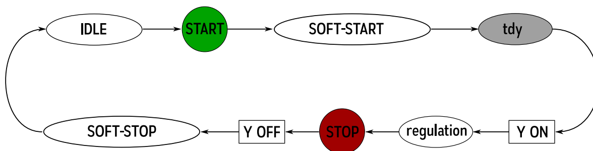
Rysunek 4: Algorytm sterowania silnikiem
